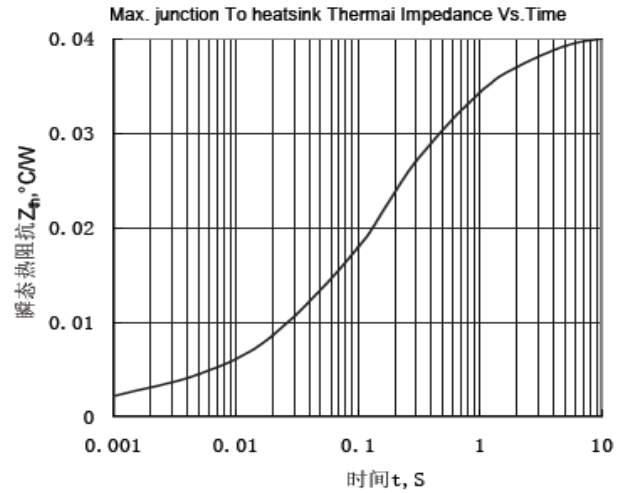
Fig.2 结至散热至瞬态热阻抗曲线
